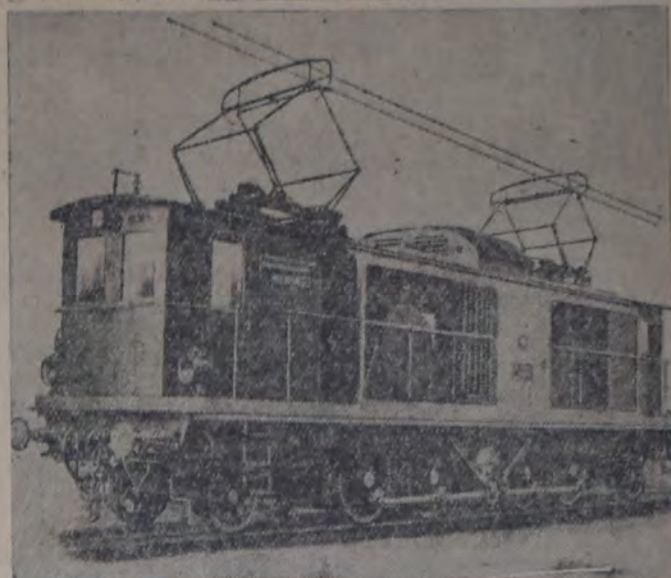
Fig. 1. — Tipo de locomotora eléctrica para trenes de mercancías y mixtos de cuatro ejes acoplados, con un eje portador delantero y otro detrás (1-D-1) de empleo generalizado. Su potencia es de 3000 H. P.
